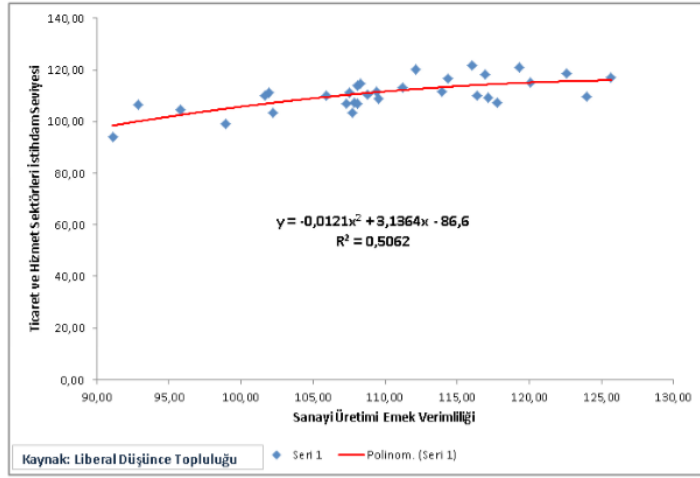
Grafik 12: Veri Dağılımı ve Regresyon
